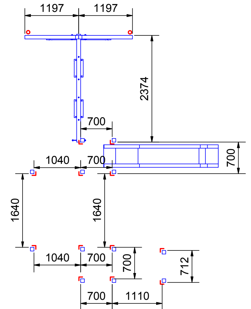
Fundamentplan mit Treppe
