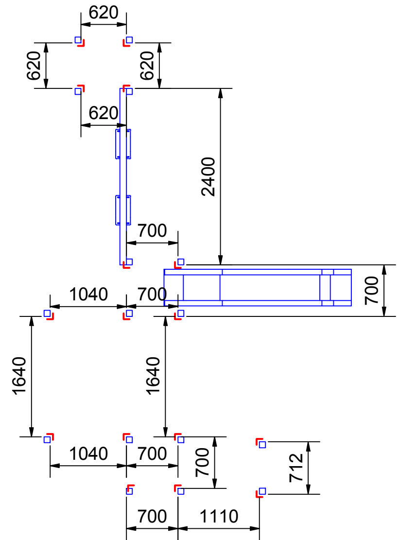
Fundamentplan mit Treppe 16 x Winkelanker
