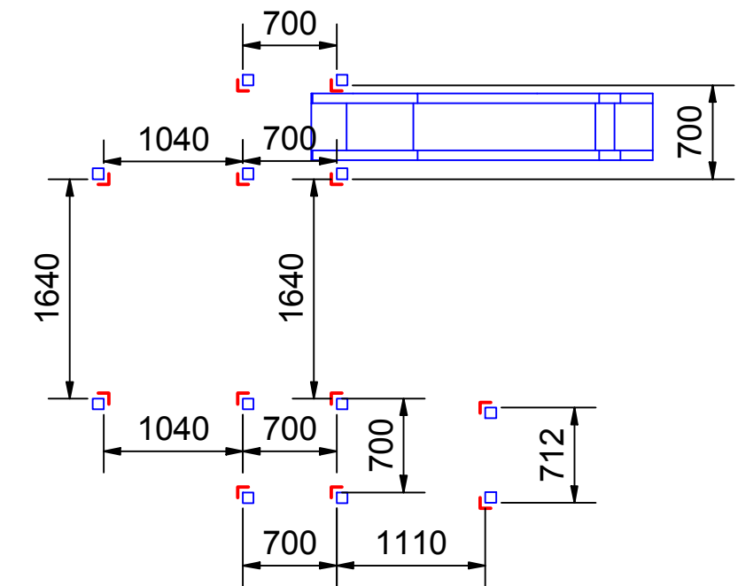
Fundamentplan mit Treppe L 12 x Winkelanker
