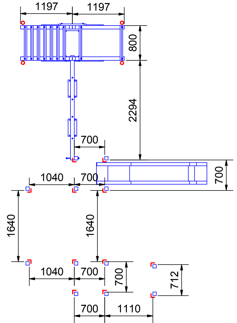
Fundamentplan mit Treppe
